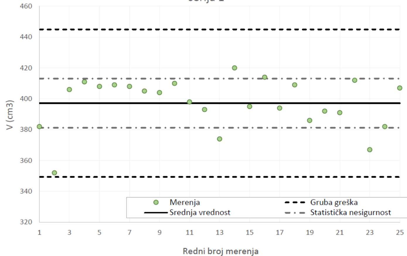
Dijagram 1.1. Merene vrednosti sa intervalom grubih grešaka - serija 1
